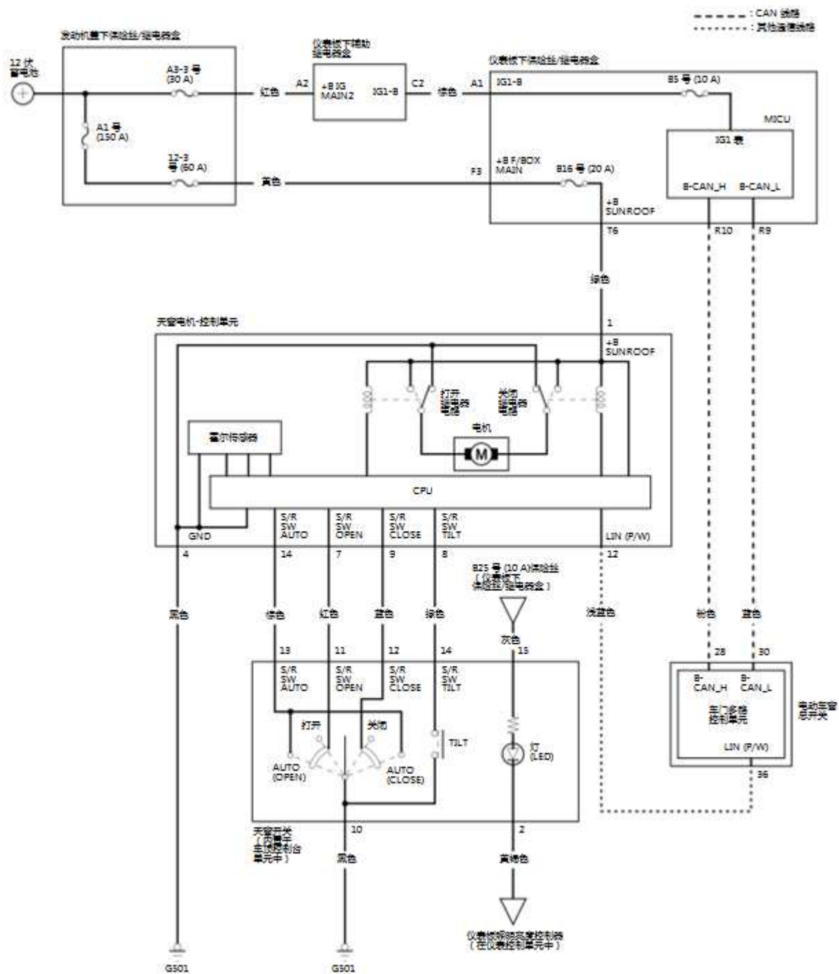
天窗电路图
